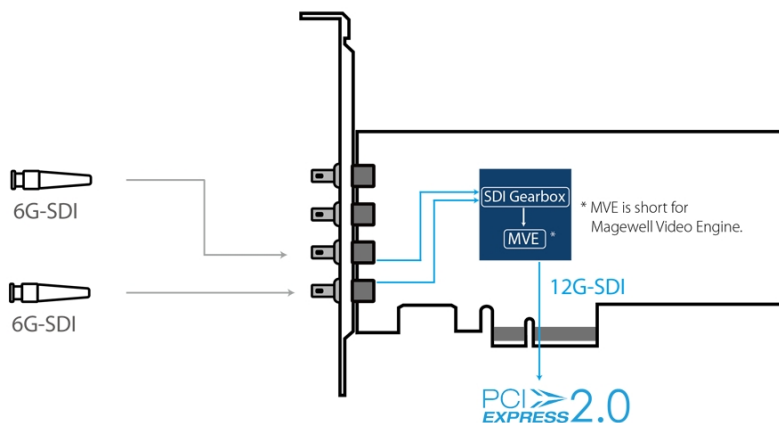
Dual-link 6G-SDI
